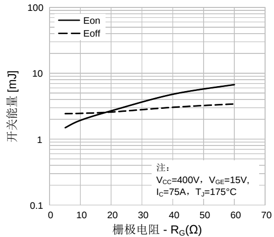
图16. 开关损耗 vs. 栅极电阻
