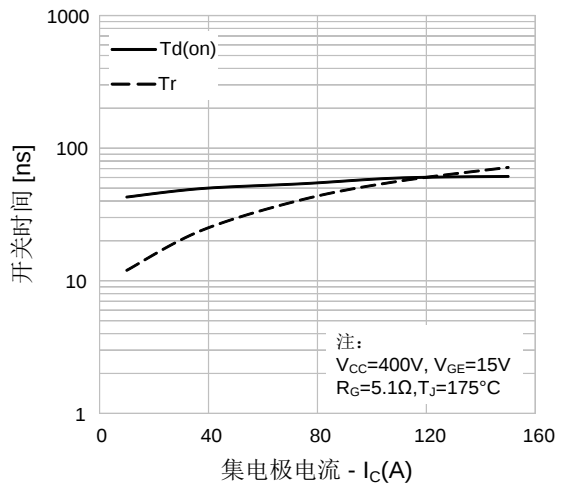
图18. 开通特性 vs. 集电极电流
