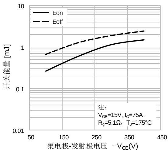
图 40. 开关损耗vs.集电极-发射极电压
