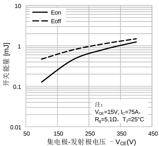
图 39. 开关损耗vs.集电极-发射极电压
