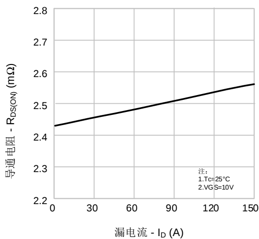
图 3. 导通电阻 vs. 漏电流
