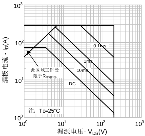
图 9-1. 最大安全工作区域(SVT20240NT/S)
