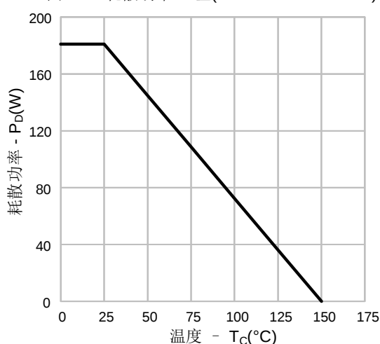
图 14-3. 耗散功率vs.温(SVSP60R160L8AD4)
