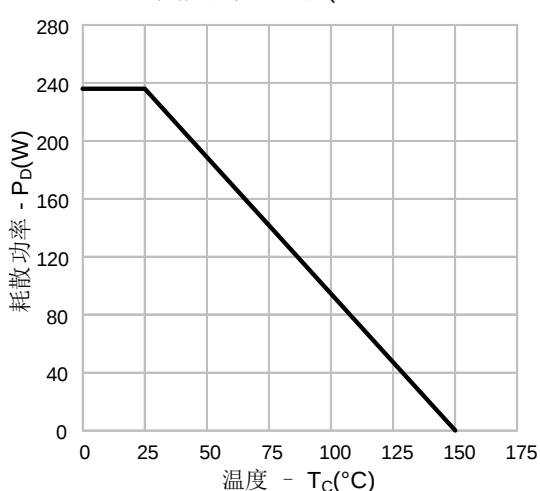
图 14-2. 耗散功率vs.温度(SVSP60R160P7D4)
