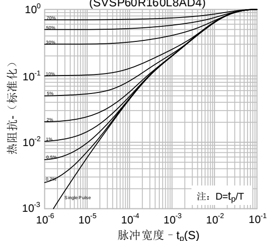
图16-3.瞬态热阻抗 vs. 脉冲宽度 (SVSP60R160L8AD4)
