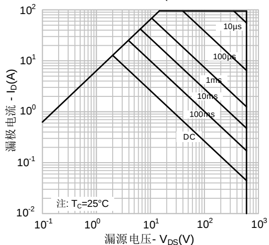
图 13-3. 最大安全工作区域(SVSP60R160L8AD4)
