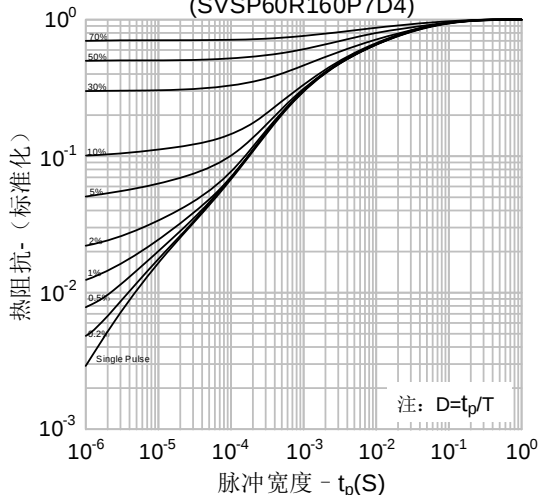
图16-2.瞬态热阻抗 vs. 脉冲宽度 (SVSP60R160P7D4)
