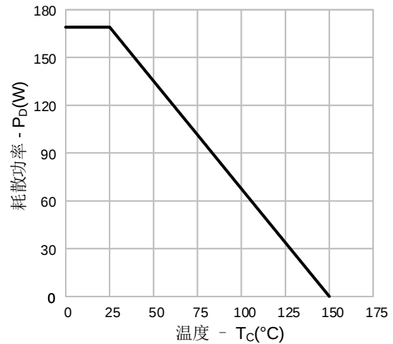
图14-3. 耗散功率vs.温度(SVSP65R180L8AD4)
