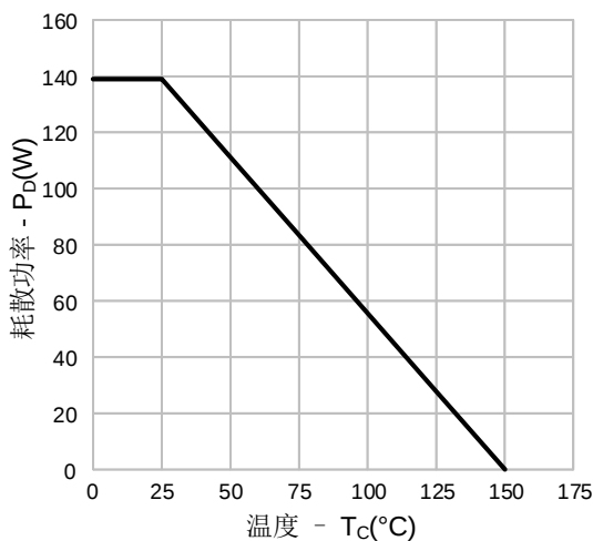
图 13-3. 耗散功率VS.温度(SVF6N90AF)
