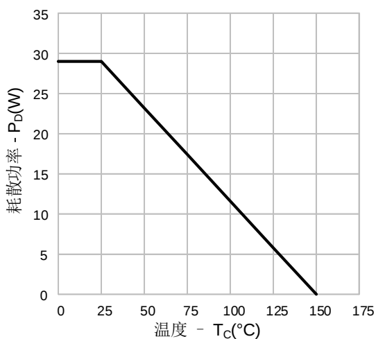
图 13-3. 耗散功率VS.温度(SVF6N90AF)
