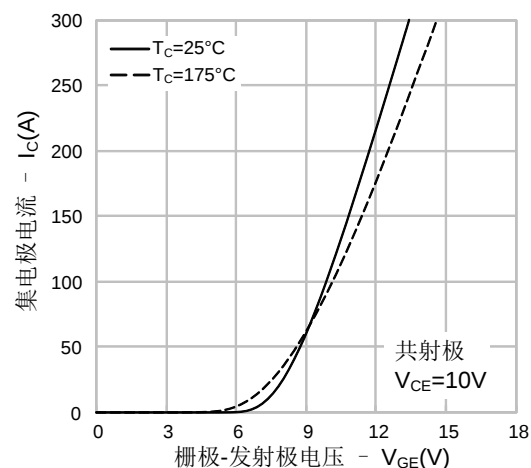
图4. 传输特性
