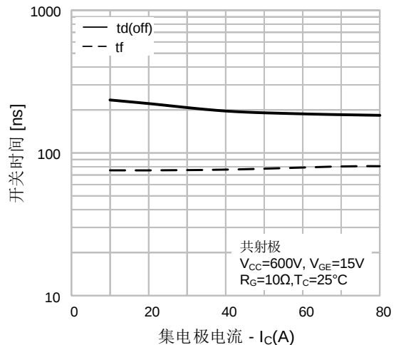
图18. 关断特性 vs. 集电极电流
