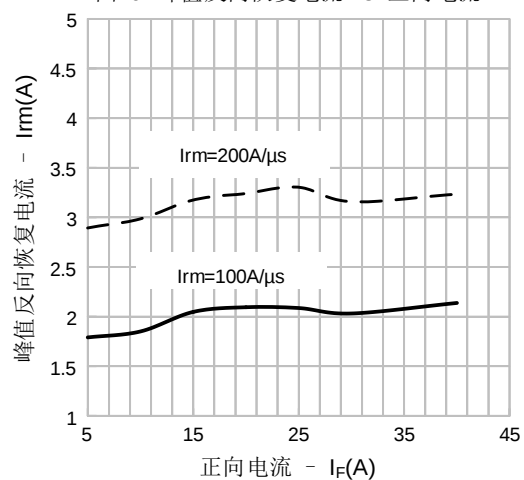
图19. 峰值反向恢复电流 vs. 正向电流
