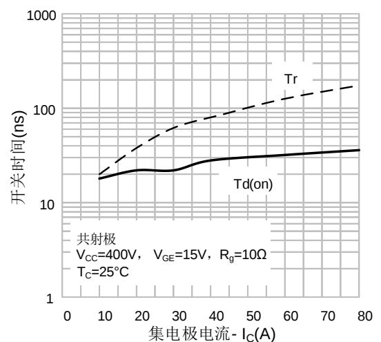
图 12. 开通特性 vs. 集电极电流
