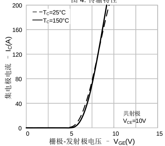
图 4. 传输特性
