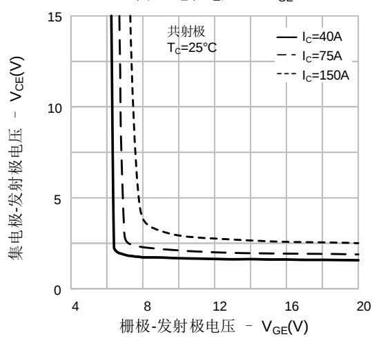
图 5. 饱和电压 vs. V_{GE}
