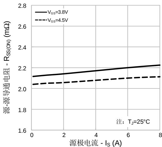
图 3. 导通电阻 vs. 源极电流
