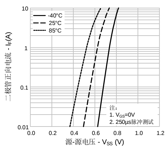
图 6. 体二极管正向压降 vs. 正向电流和温度
