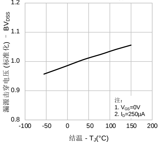
图 9. 击穿电压 vs. 温度特性
