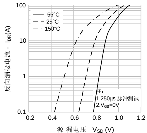
图 4. 体二极管正向压降 vs. 源极电流和温度
