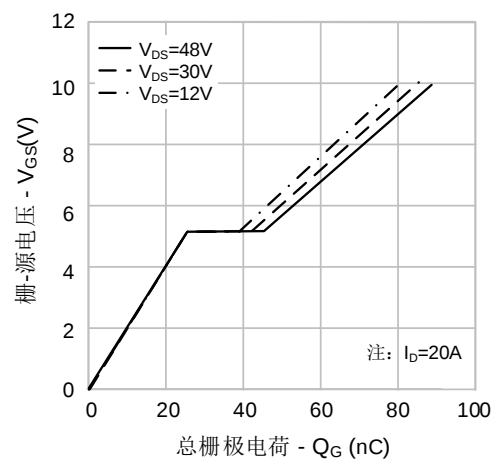
图 6. 电荷量特性
