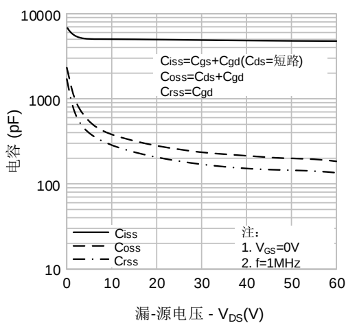
图 5. 电容特性
