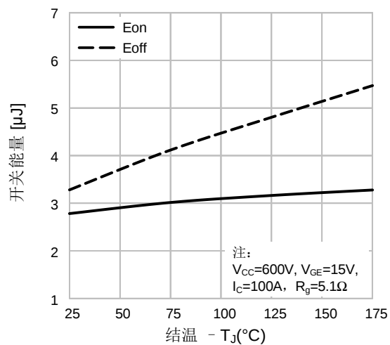
图 38. 开关损耗vs.温度特性
