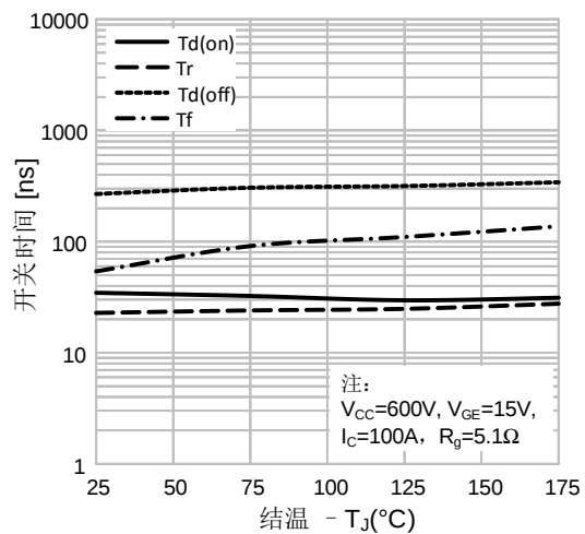
图 37. 开关时间vs.温度特性
