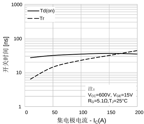
图17. 开通特性 vs. 集电极电流
