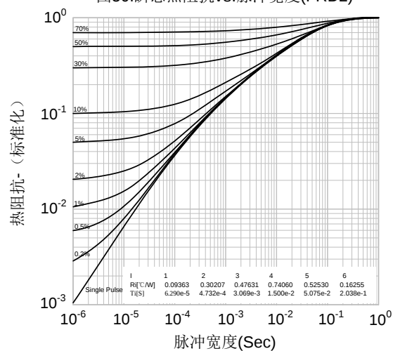
图50.瞬态热阻抗vs.脉冲宽度(FRD2)
