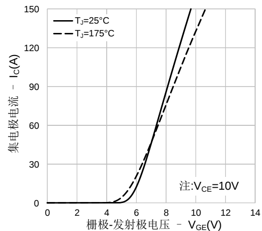
图4. 传输特性
