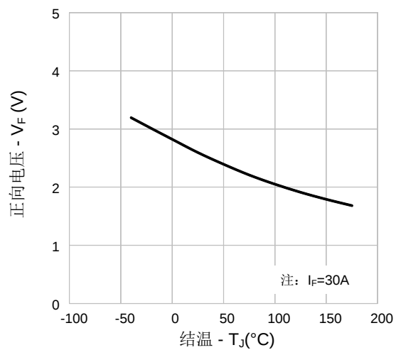
图49.二极管正向电压vs.温度特性(FRD2)
