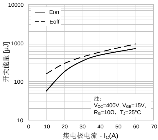
图21. 开关损耗 vs. 集电极电流
