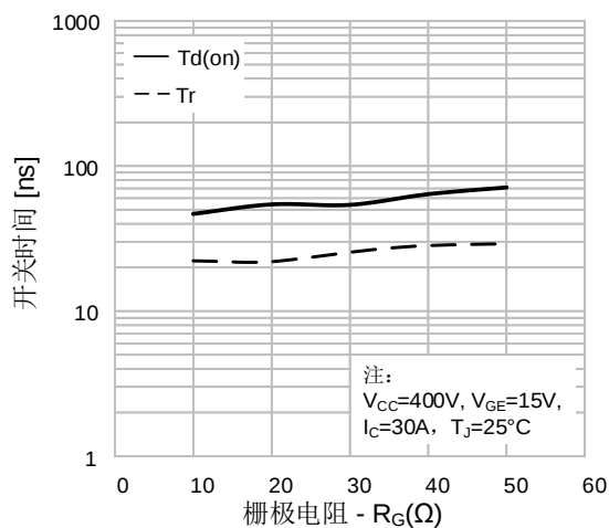
图11. 开通特性 vs. 栅极电阻
