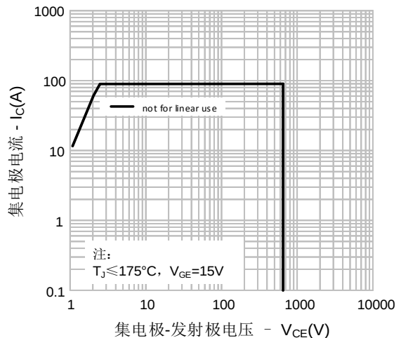
图 30. 安全工作区
