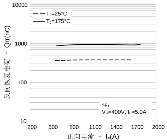
图 24. 反向恢复电荷 vs. 正向电流
