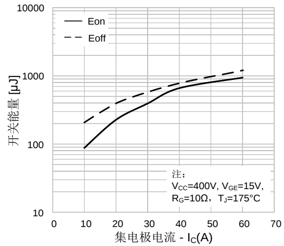
图22. 开关损耗 vs. 集电极电流
