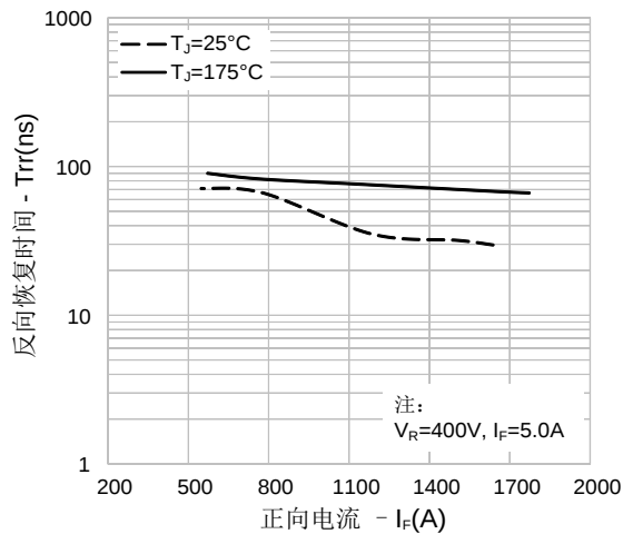
图23. 反向恢复时间 vs. 正向电流
