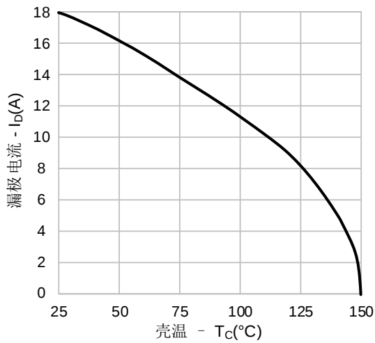
图13. 最大漏电流vs. 壳温
