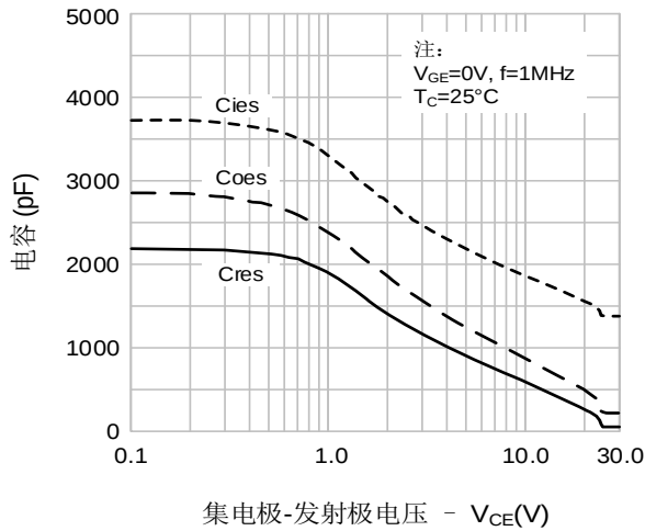
图7. 电容特性
