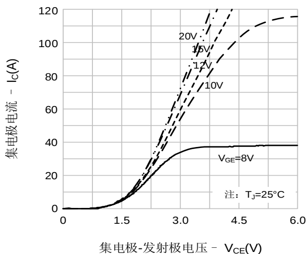
图1. 典型输出特性
