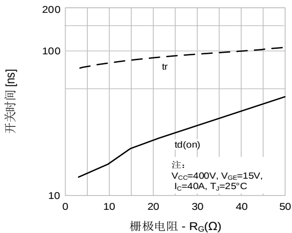
图9. 开通特性 vs. 栅极电阻
