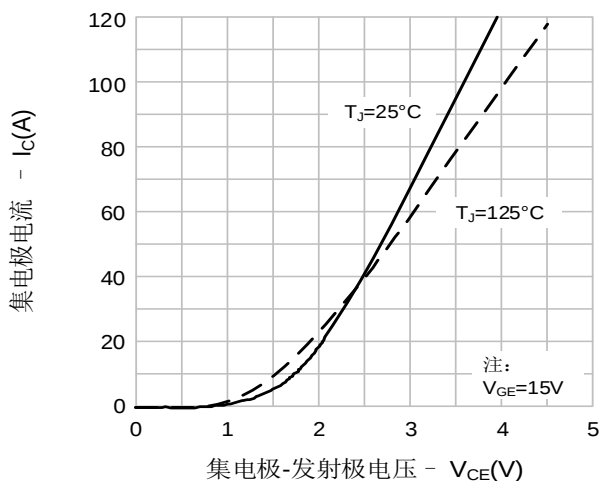
图3. 典型饱和电压特性
