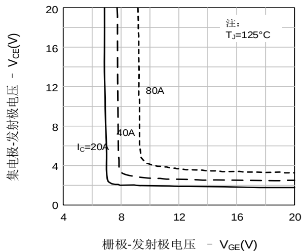
图6. 饱和电压 vs. V_{GE}
