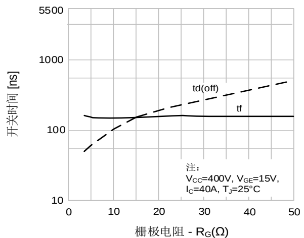
图10. 关断特性 vs. 栅极电阻
