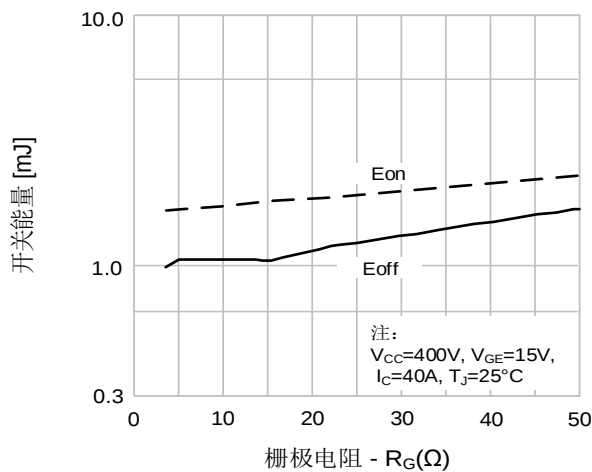
图11. 开关特性 vs. 栅极电阻
