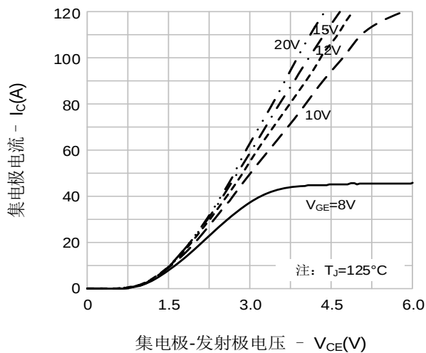
图2. 典型输出特性
