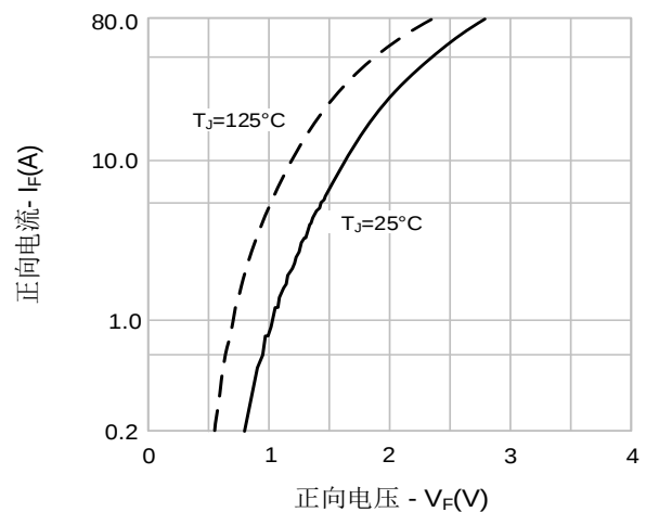
图12. 正向特性
