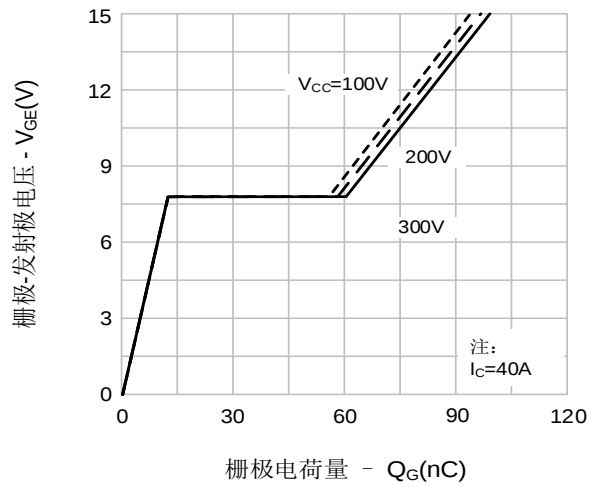
图8. 栅极电荷特性
