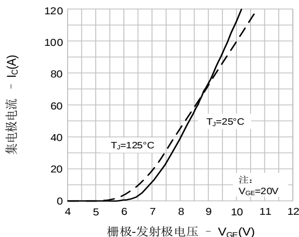
图4. 传输特性
