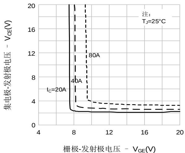
图5. 饱和电压 vs. V_{GE}
