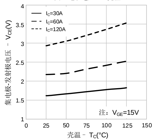
图6. 饱和电压 vs. 壳温
