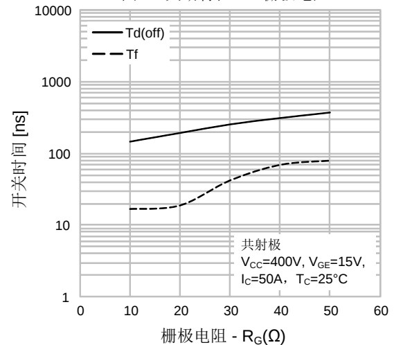
图12. 关断特性 vs. 栅极电阻
