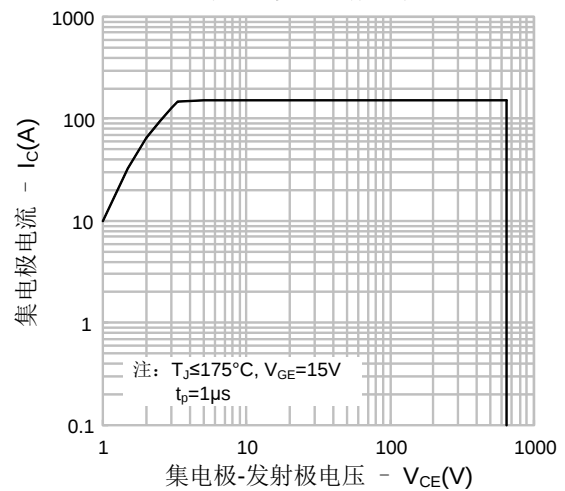
图22. 安全工作区域
