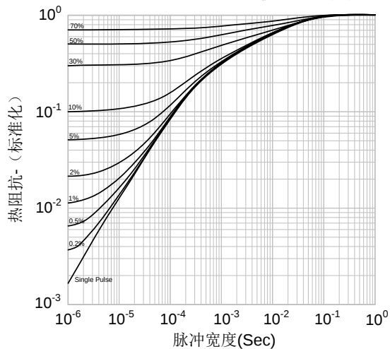
图23. IGBT 瞬态热阻抗vs.脉冲宽度
