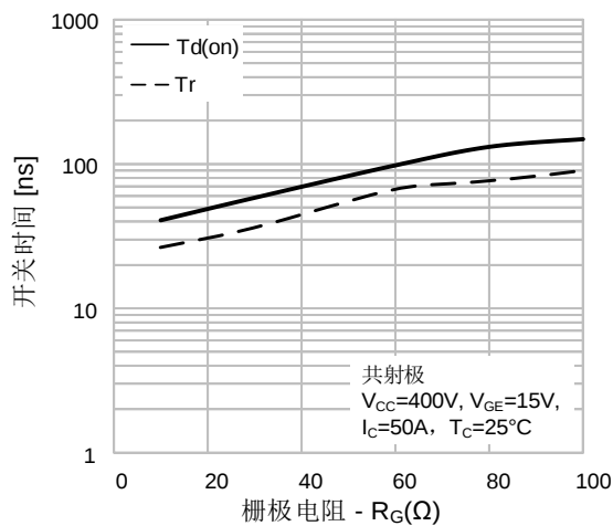
图11. 导通特性 vs. 栅极电阻
