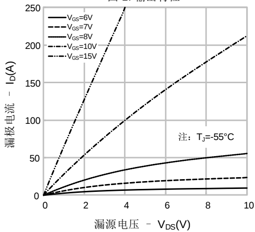
图 3. 输出特性
