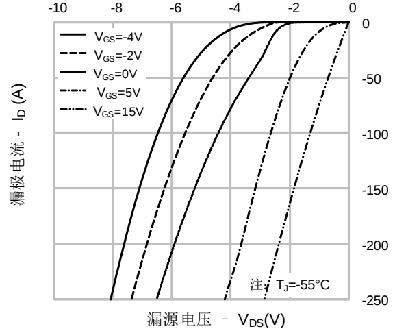
图 10. 体二极管正向压降 vs. 源极电流
