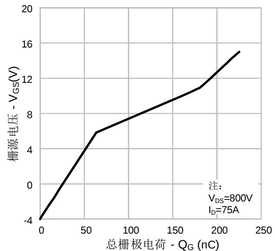
图 12. 电荷量特性
