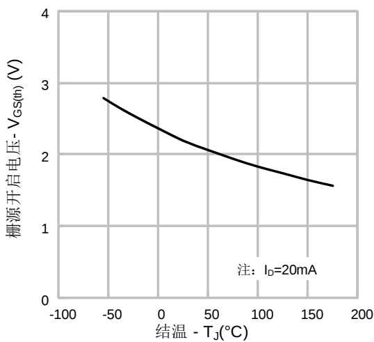
图 11. 开启电压 vs. 温度特性
