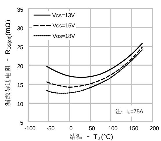
图 6. 导通电阻vs.结温
