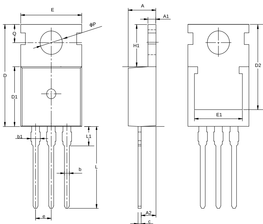
TO-220A-3L
