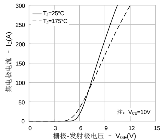
图4. 传输特性
