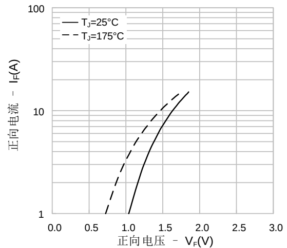
图 10. 正向特性
