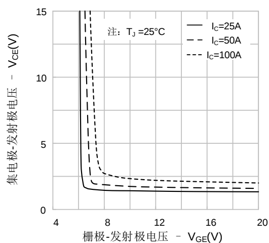
图5. 饱和电压 vs. Vge
