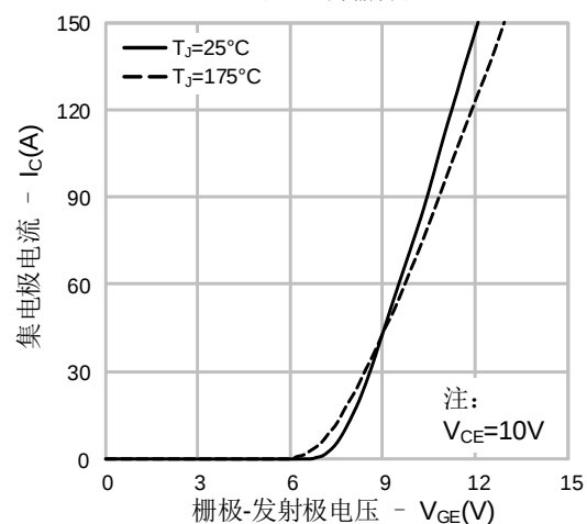
图4. 传输特性
