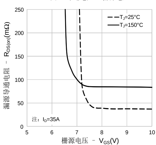
图 6. 导通电阻vs.栅源电压
