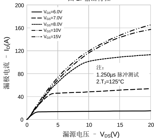
图 2. 输出特性
