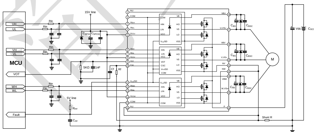
7.典型应用电路图
