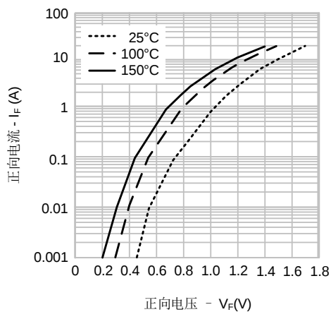
图1. 正向特性
