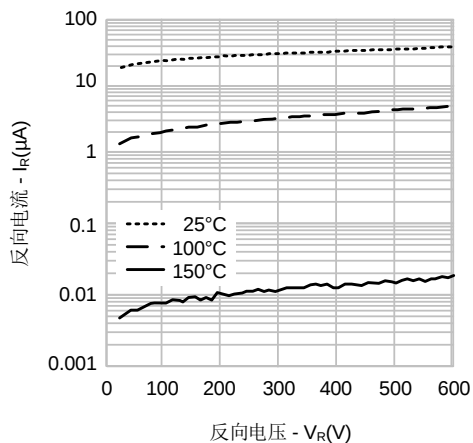
图3. 反向特性
