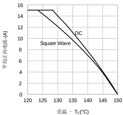
图5. 正向电流降额曲线
