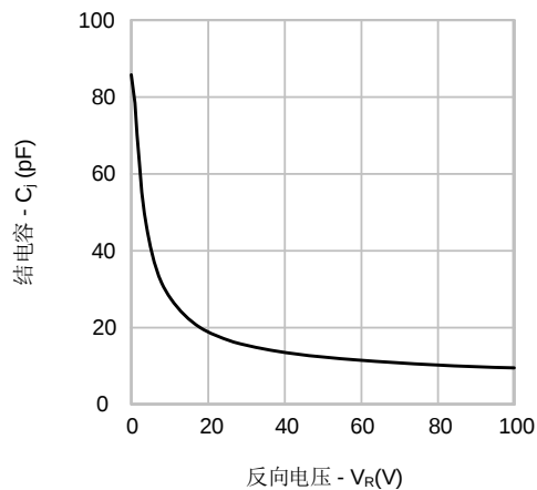
图2. 结电容特性
