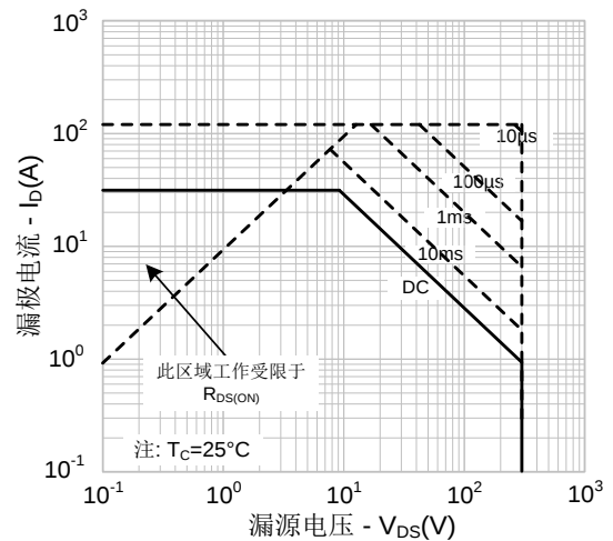
图13. 最大安全工作区域
