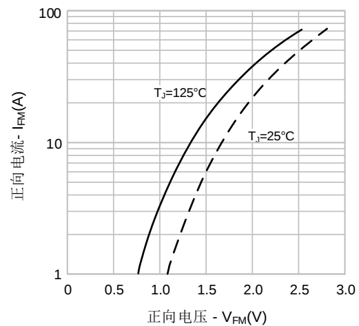
图16. 正向特性
