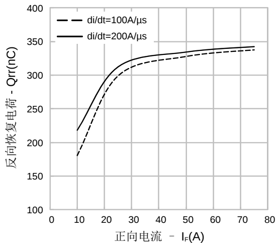
图 24. 反向恢复电荷 vs. 正向电流
