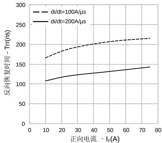
图23. 反向恢复时间 vs. 正向电流
