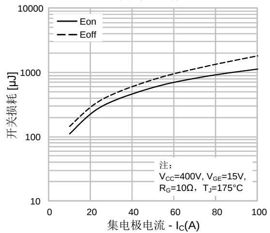
图22. 关断损耗 vs. 集电极电流
