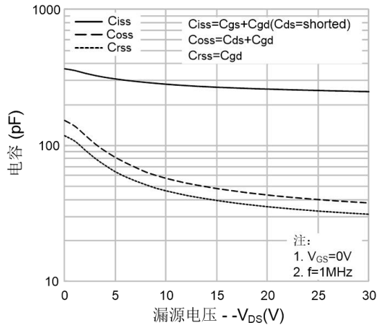
图7. 电容特性
