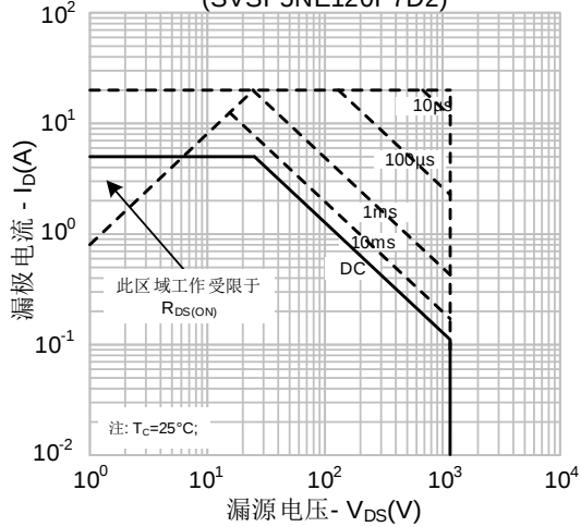
图 13-3. 最大安全工作区域 (SVSP5NE120FJDD2)
