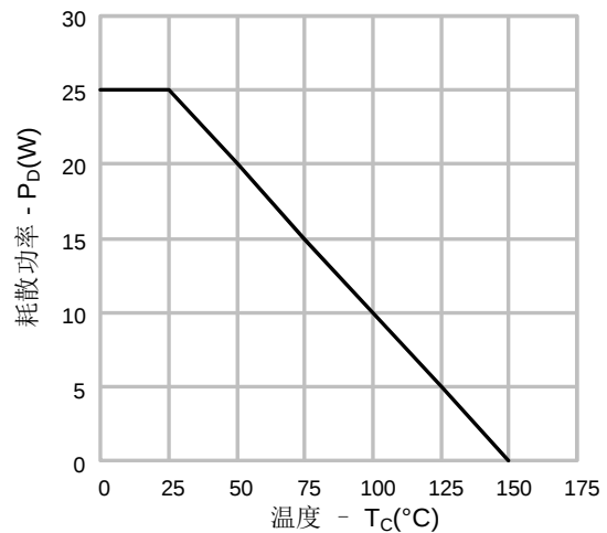
图14-3. 耗散功率vs.温度(SVSP5NE120FJDD2)
