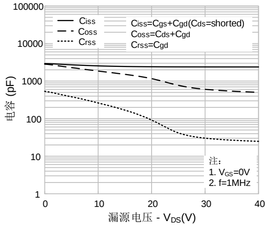
图7. 电容特性
