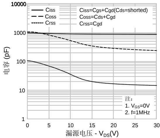
图7. 电容特性
