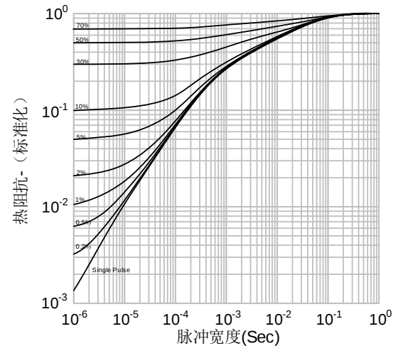
图30. 二极管瞬态热阻抗vs.脉冲宽度
