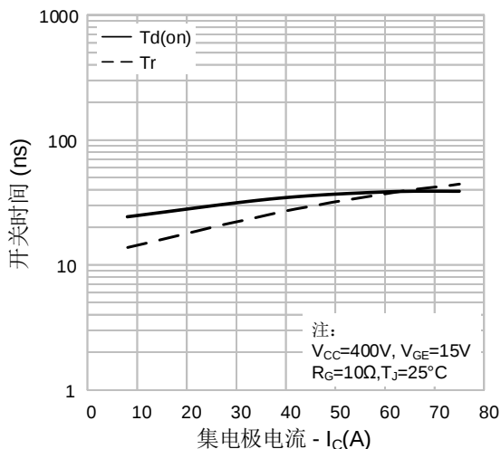
图17. 开通特性 vs. 集电极电流
