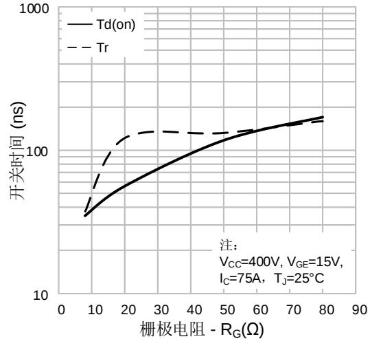
图11. 开通特性 vs. 栅极电阻
