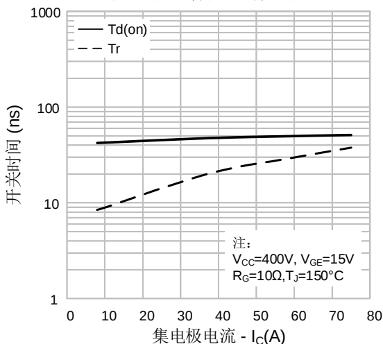
图18. 开通特性 vs. 集电极电流
