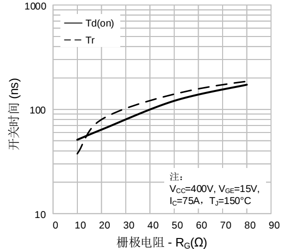
图12. 开通特性 vs. 栅极电阻
