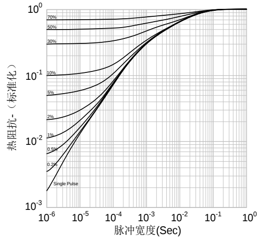
图28. IGBT 瞬态热阻抗vs.脉冲宽度
