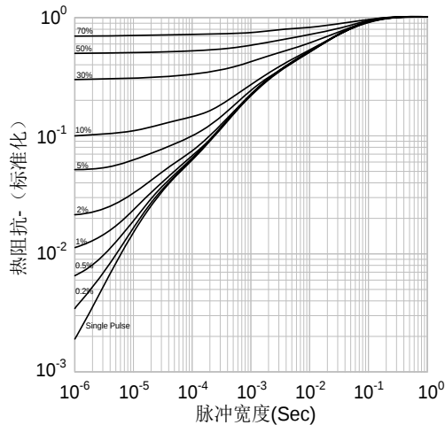
图29.二极管瞬态热阻抗vs.脉冲宽度
