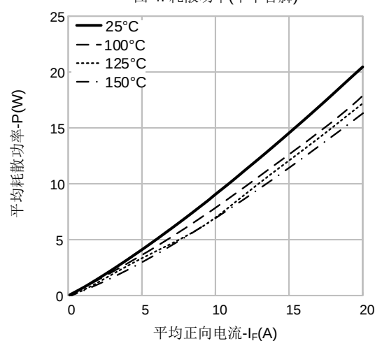
图 4. 耗散功率(单个管脚)
