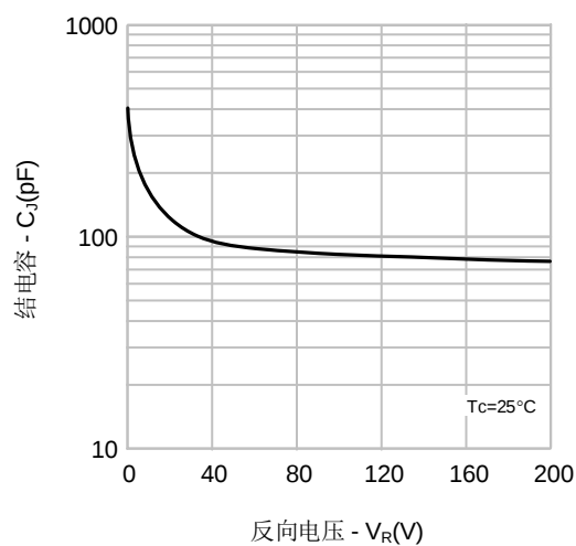
图 4. 结电容特性
