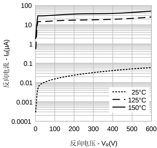
图3. 反向特性
