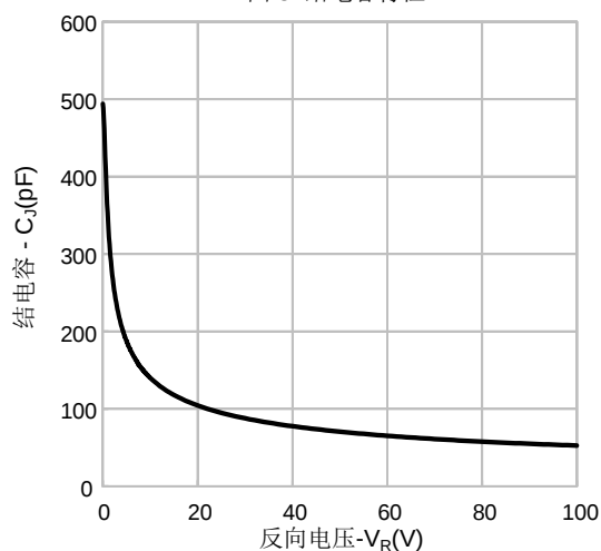
图 3. 结电容特性
