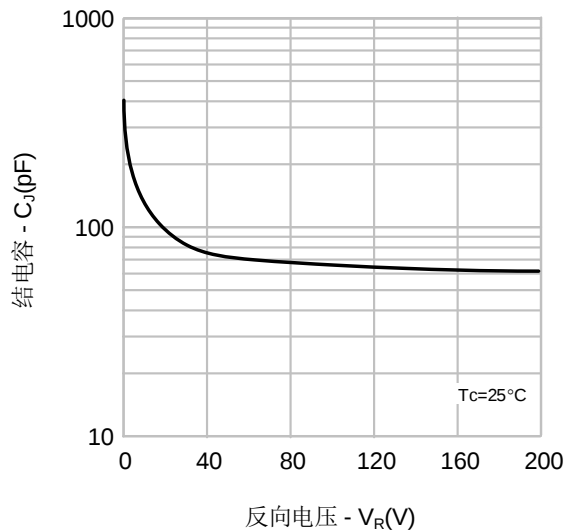
图 4. 结电容特性
