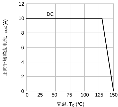
图5. 正向平均电流降额曲线
