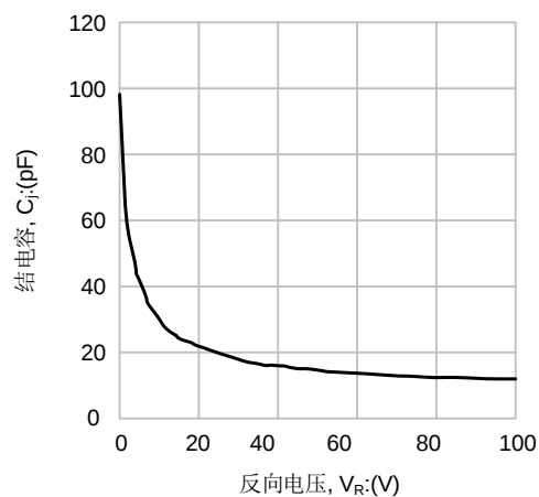
图2. 结电容特性
