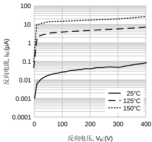
图3. 反向特性
