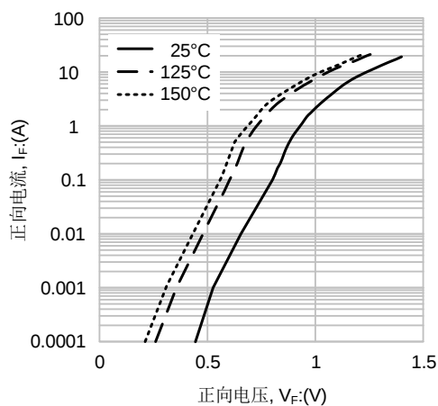
图1. 正向特性
