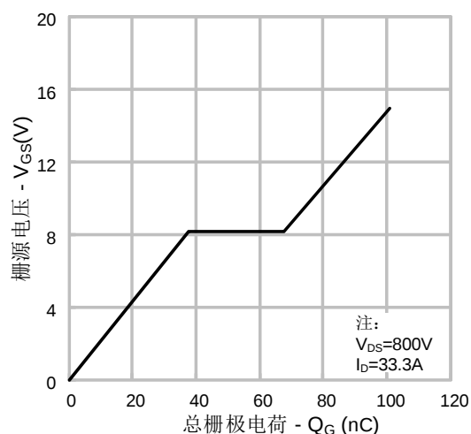
图 12. 电荷量特性
